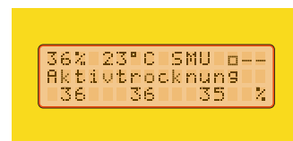
Mit zwei Efidry-Sensoren erfasst die DA 4 Qube gleichermaßen Mischungsverhältnis und relative Feuchtigkeit der Prozessluft sowie zusätzlich Raumluftfeuchte und -temperatur. Alle Statusinformationen werden Ihnen im Wechsel als „Klartext“ auf dem beleuchteten Dreizeilendisplay der DA 4 Qube angezeigt.
