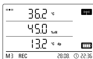
Ejemplo de visualización de una incidencia de alarma del canal de medición representado en la primera línea de valores de medición.
